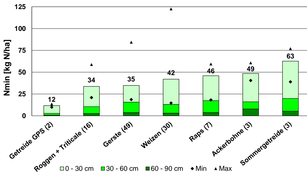
Abb. 1: Durchschnittliche Ernte-Nmin Ergebnisse nach Hauptfrüchten 2020
