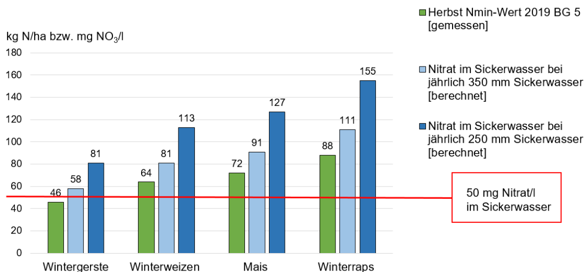
Abb. 3: Nitrat im Sickerwasser in Abhängigkeit des Herbst-Nmin-Wertes 2019 und der Sickerwasserraten im BG 5
